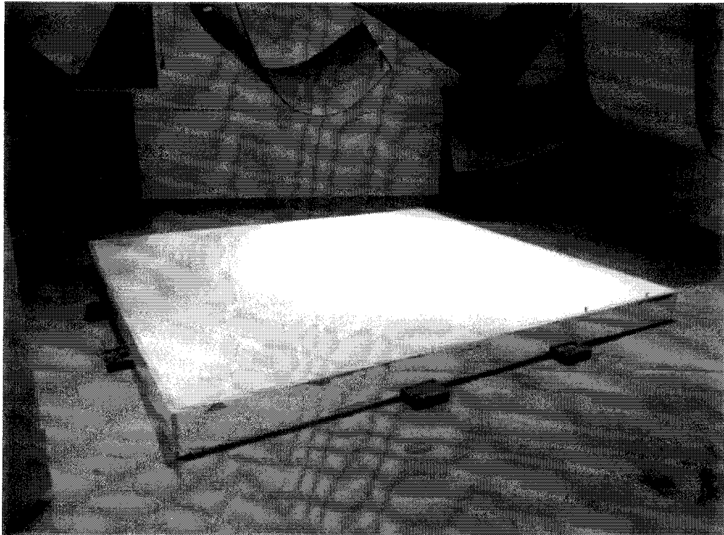
Abb. 2 : Ansicht Prüfaufbau im Hallraum
