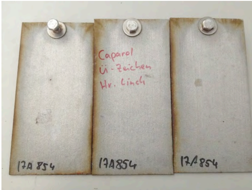
Bild 1 – Gestrahlte Stahlbleche (SA2,5) / Capalac Dickschichtlack Glimmer RAL 9007 nach 5 Jahren Freibewitterung
